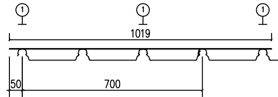
Klip-Lok 700 SMD300M-6X10UW
