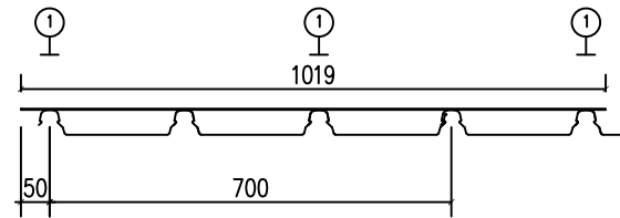
Klip-Lok 700 SMD360M-6X12UW
