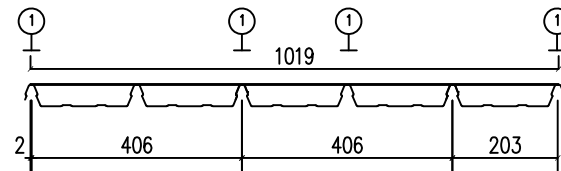
Klip-Lok 406 SMD300M-6X10UW
